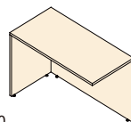
N145L/R W1200*D600*H745 W890*D600*H745 W766*D600*H745
