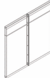
直线连接系统 Straight connection
